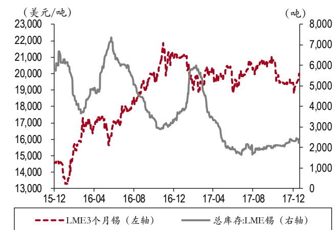
图表 21. LME 3 个月锡价格高位震荡、库存企稳
