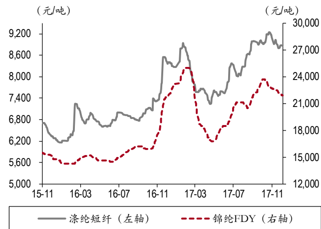
图表 39. 化纤: 涤纶短纤回升, 锦纶继续回落
