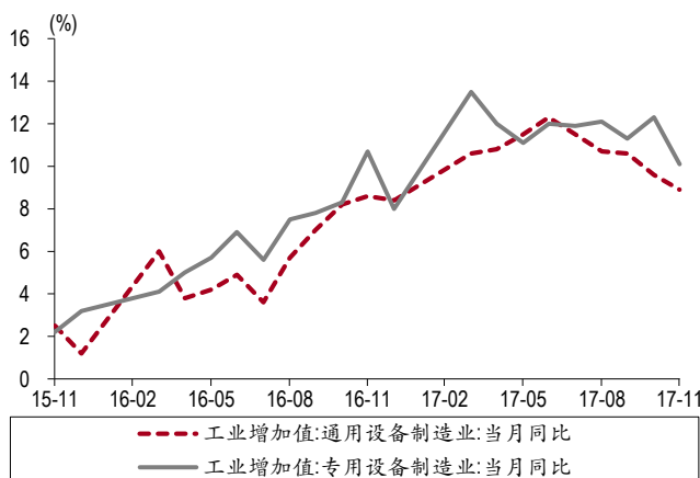
图表 45. 机械设备 11 月工业增加值增速下滑
