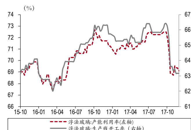
图表 34. 浮法玻璃产能利用率低位震荡
