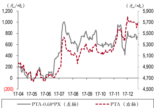
图表 36. PTA-PX 价差高位震荡
