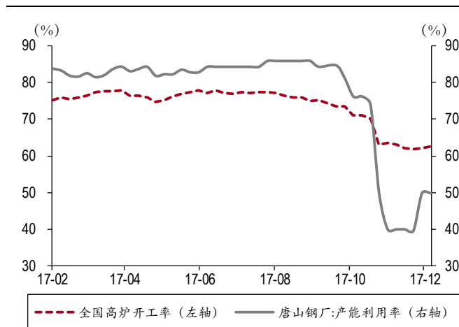
图表 29. 产能利用率大幅回升
